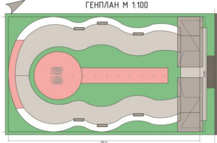
ГЕНПЛАН М 1:100
